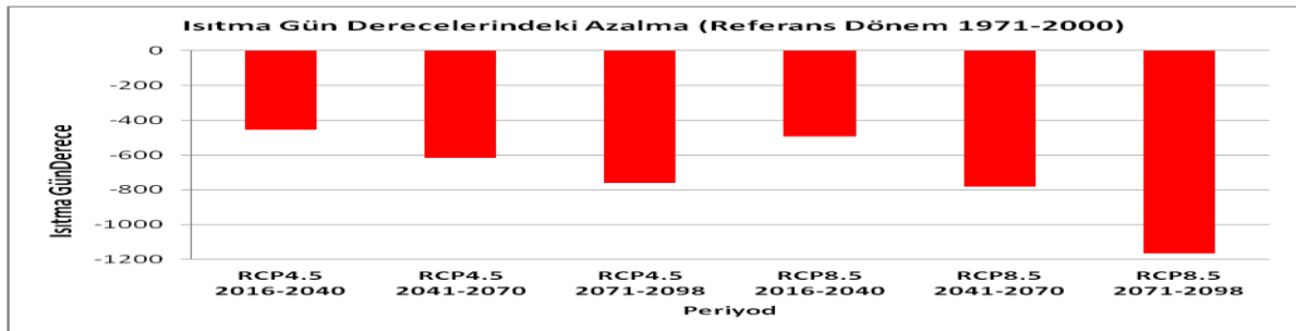
Grafik 2: HadGEM2-ES modeli gelecek dönemler yıllık Isıtma Gün Dereceleriindeki azalma
